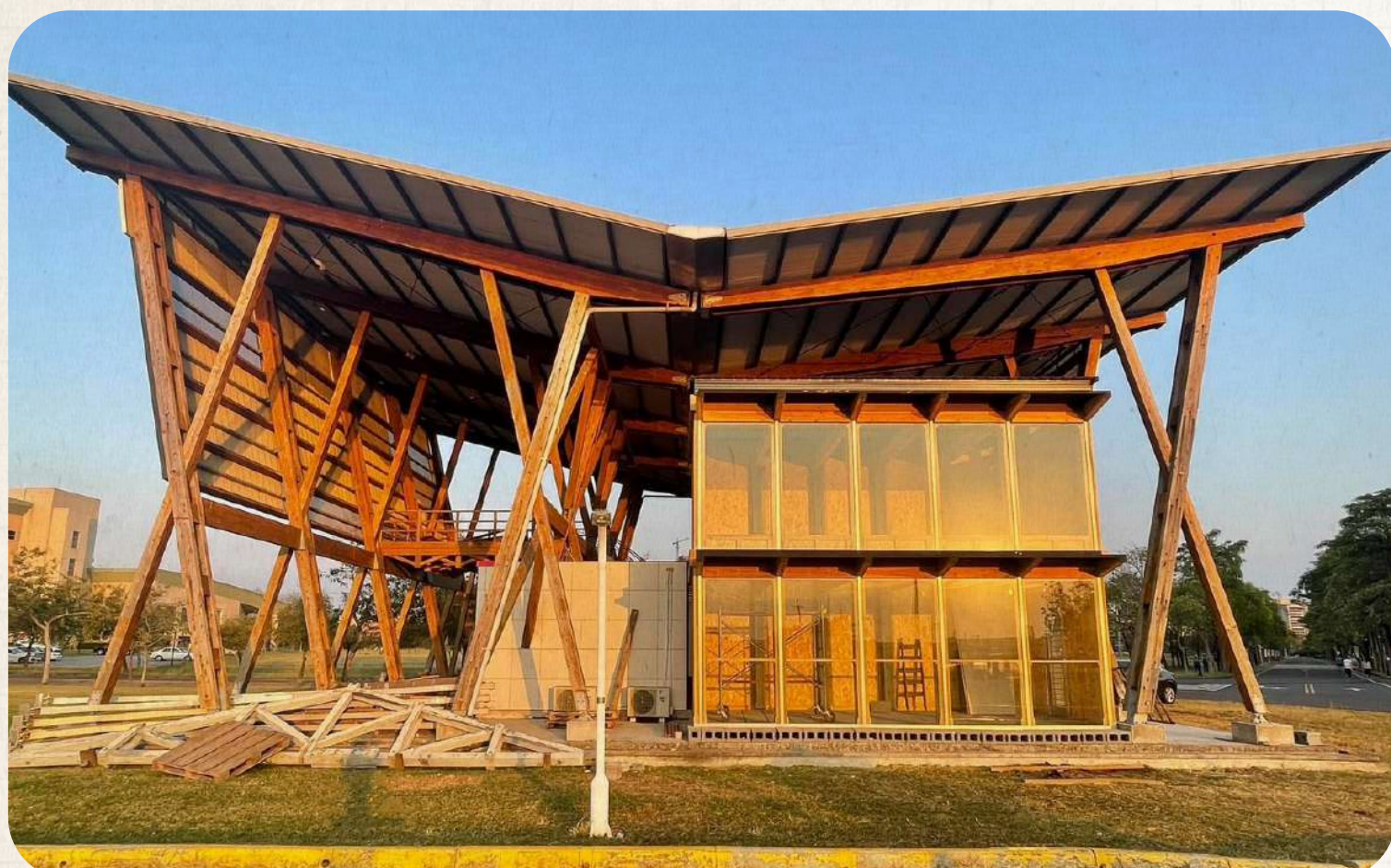
本系陳啓仁教授主持國立高雄大學木構造實驗示範屋 (Demo Building)
